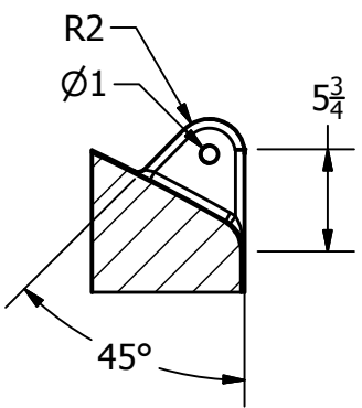
SECTION A-A SCALE 1:12
